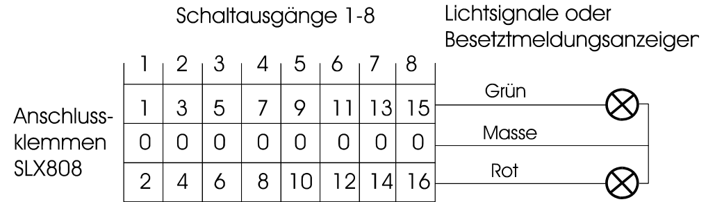
Anschluss Lichtsignale oder Besetztanzeige
